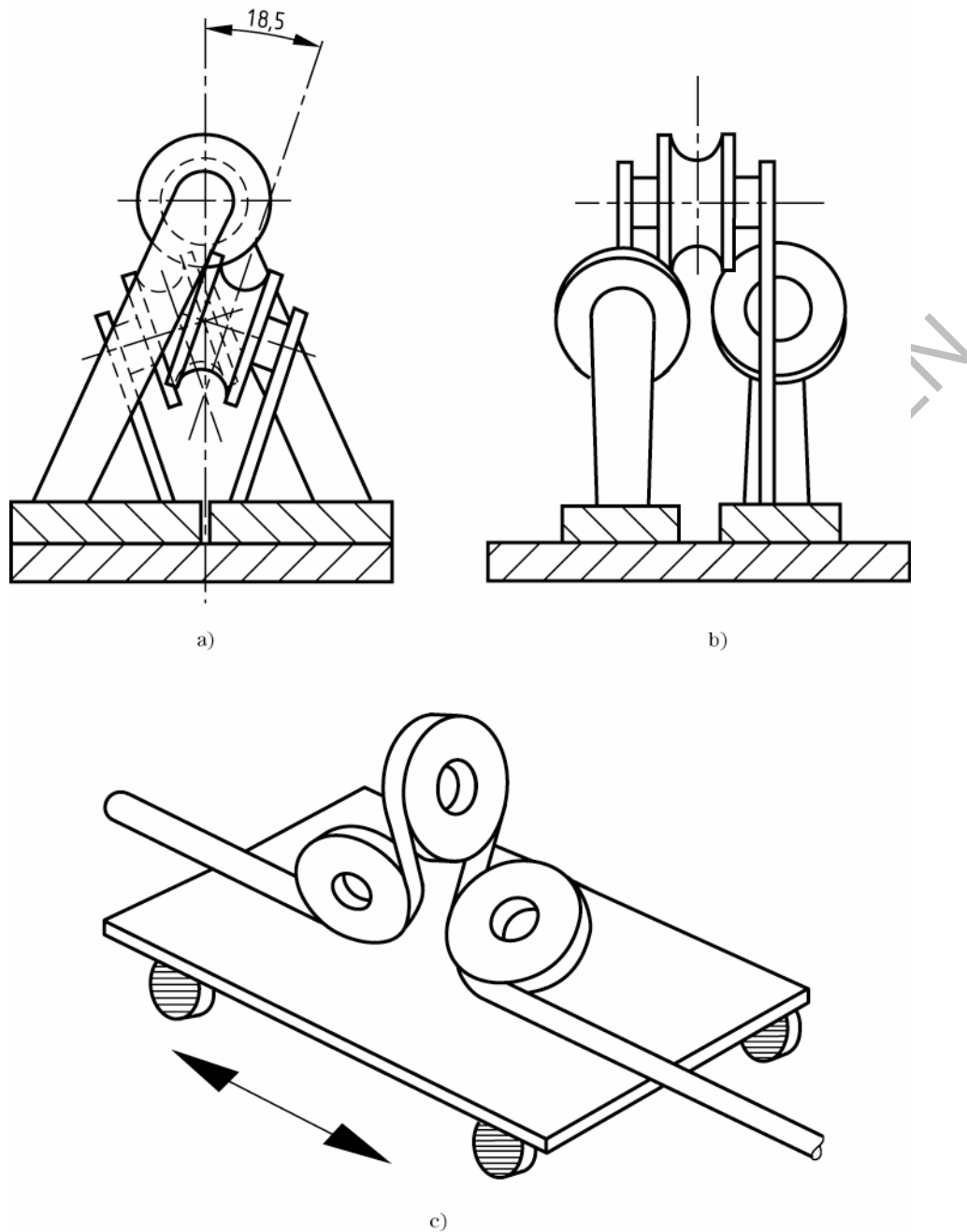
Figure 5 - Chariot "C" modifié
